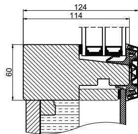
Fuldisoleret fylding med eternit panel udvendig
