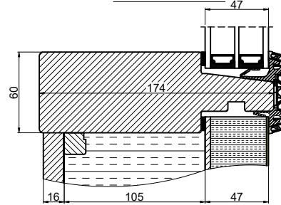
Fuldisoleret fylding med glat fylding udvendig 184 mm karm
