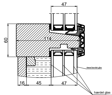
Fuldisoleret fylding med emalit glas udvendig
