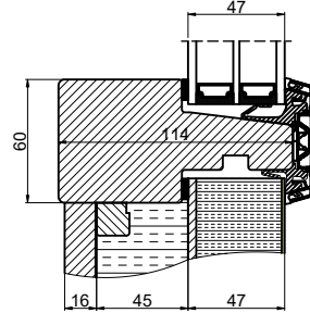
Fuldisoleret fylding med glat fylding udvendig
